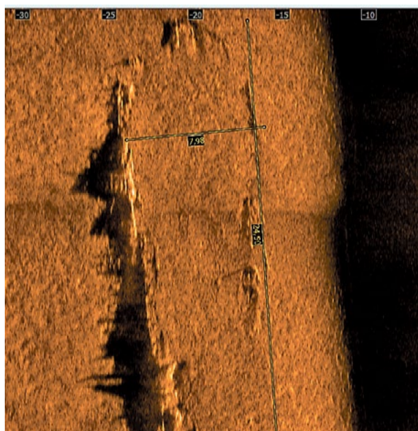
Изображения кораблей были получены с помощью гидролокаторов, то есть звука. Таким образом, это, по сути, псевдоизображения, каждая точка которых показывает, как громко откликнулся объект
